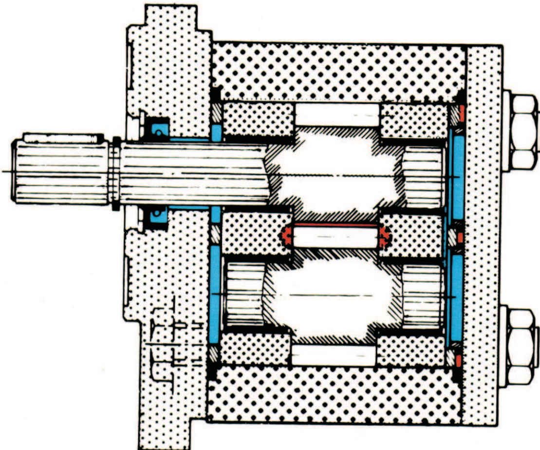
pompe à engrenages à denture externe
