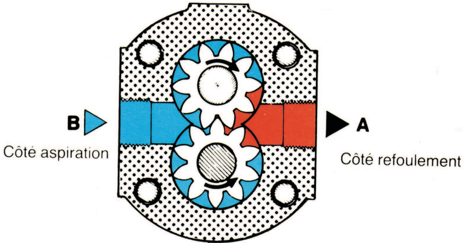
pompe à engrenages à denture externe
